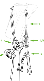
4.4 Kambiumschoner für Einfachseil abgeknotet Cambium saver for single rope, knotted
