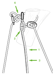
4.5 Kambiumschoner für Einfachseil als Würgeschlinge Cambium saver for single rope as choke sling
