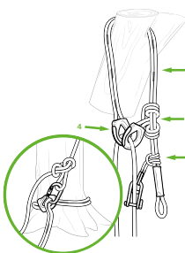
4.3 Kambiumschoner für Einfachseil mit Anschlagpunkt am Stamm Cambium saver for single rope with anchor point on tree trunk
